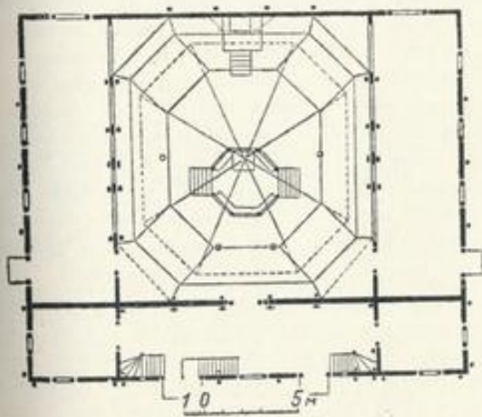
31. План деревянной синагоги
