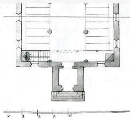
Разрез и план лютеранской церкви св. Иоанна в Гродно. 1840 г. Ф. 1488. Оп. 1. Д. 947. Л. 1
