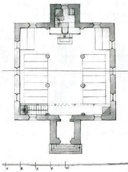
Разрез и план лютеранской церкви св. Иоанна в Гродно. 1840 г. Ф. 1488. Оп. 1. Д. 947. Л. 1
